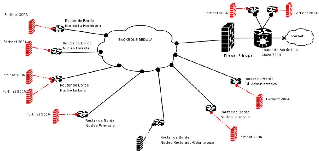
PROPUESTA DE ARQUITECTURA DE SEGURIDAD PARA ReDULA
